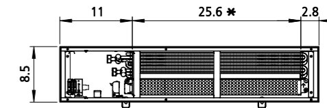
Raumseite / Room side
