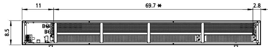
Raumseite / Room side
