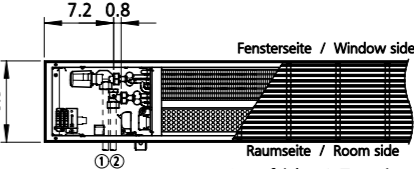
Draufsicht / Top view
