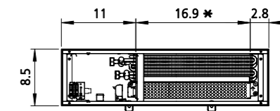
Raumseite / Room side
