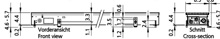
Vorderansicht / Front view
